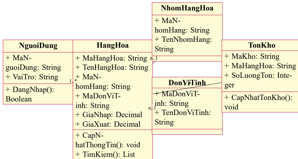
Hình 4.4: Biểu đồ lớp trong ca sử dụng UC05 – Quản lý hàng hóa
